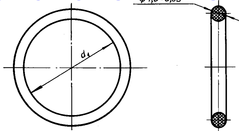
Размеры, мм
