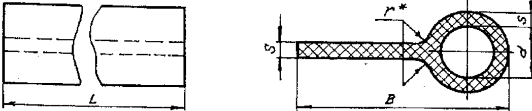
Размеры, мм
