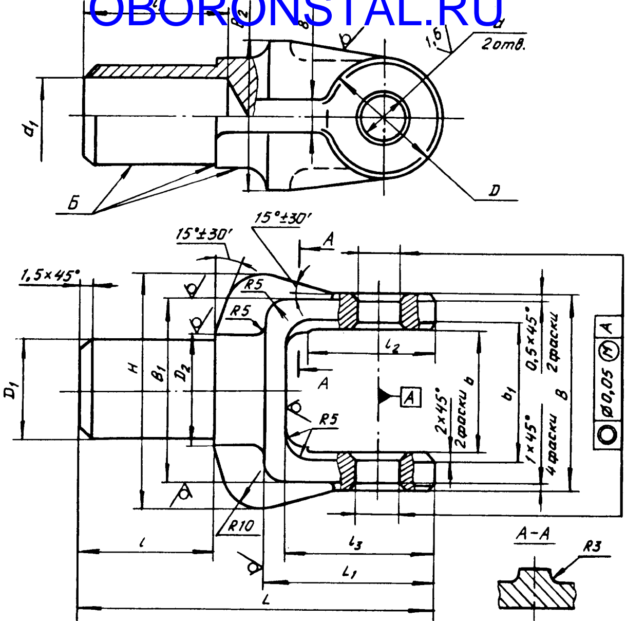
Размеры, мм
