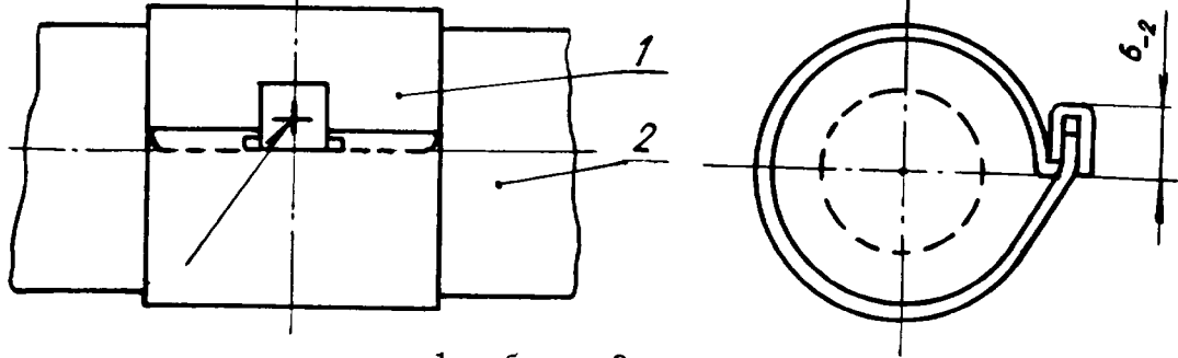
1 - бирка; 2 - рукав
