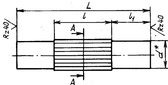
Размеры, мм
